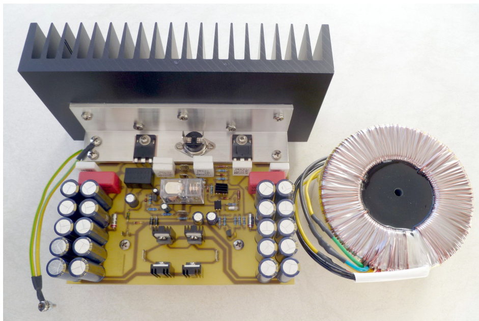
SE 25 Modul mit vergossenem 225 VA Ringkerntrafo
