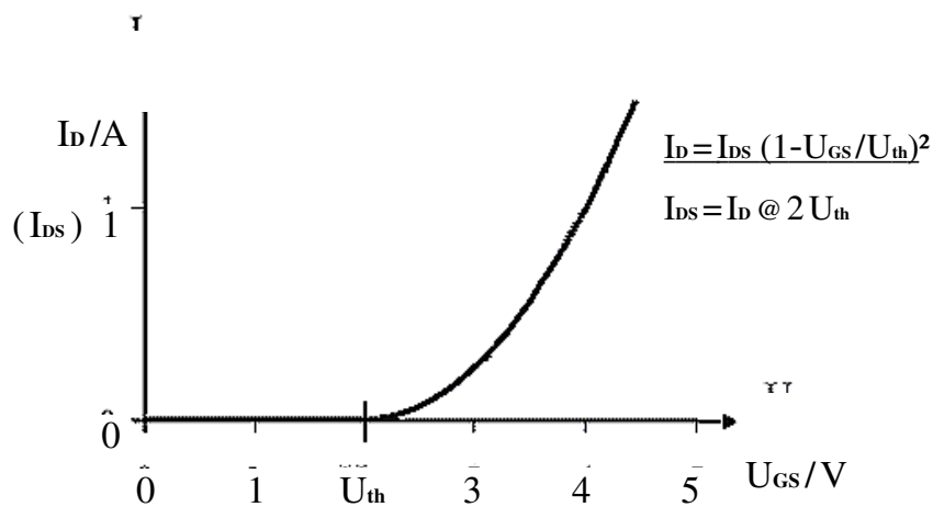
Fig. 3 Kennlinie eines MOSFET
