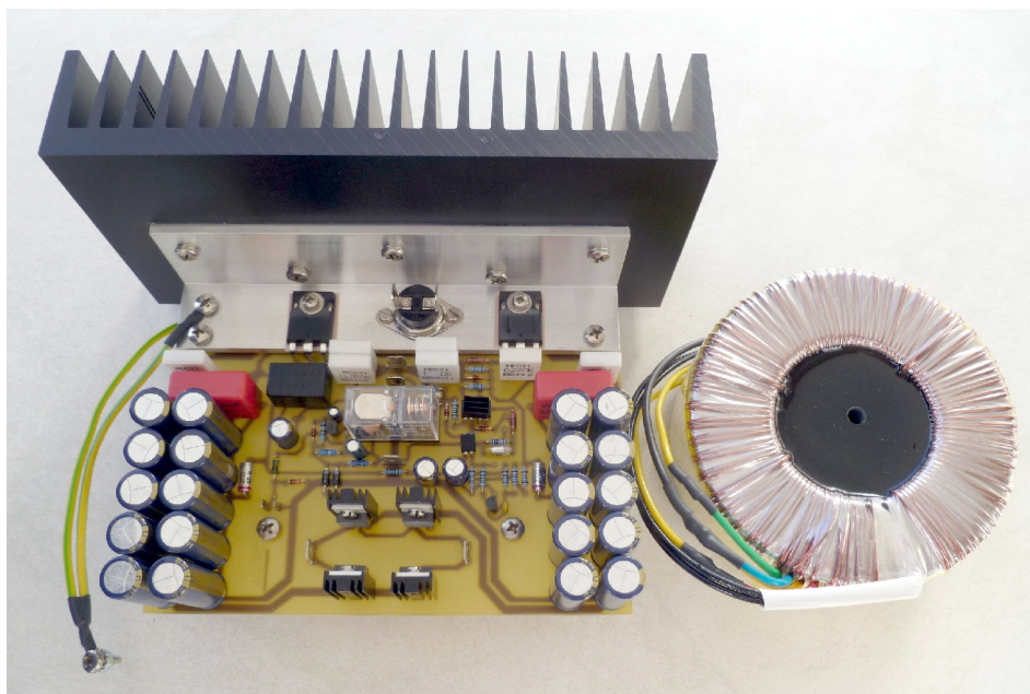
SE 25 Modul mit vergossenem 225 VA Ringkertrafo
