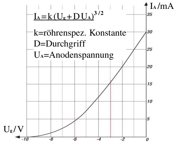
Fig. 1 Kennlinie einer Triode
